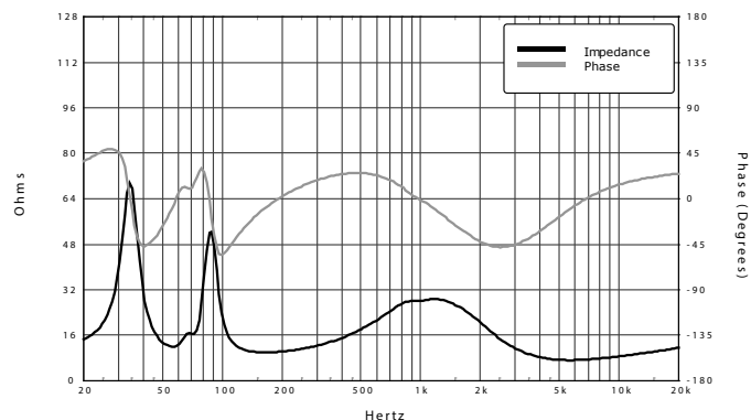
Impedance/Phase
