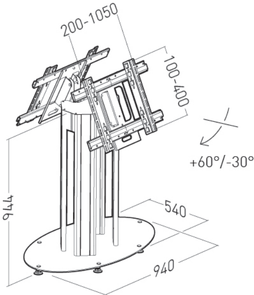
FIXE / FREESTAND
