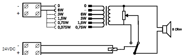
Diagramme électrique
