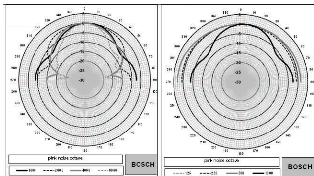
Diagrammes polaires
