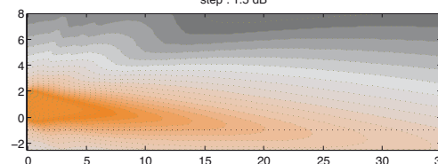
Step Array SA230P+ directivité verticale : niveau sonore pour les octaves de la parole (500Hz-1kHz-2kHz) dans le plan vertical médian.
